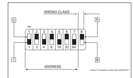
Fig. 4- DIL Switch
