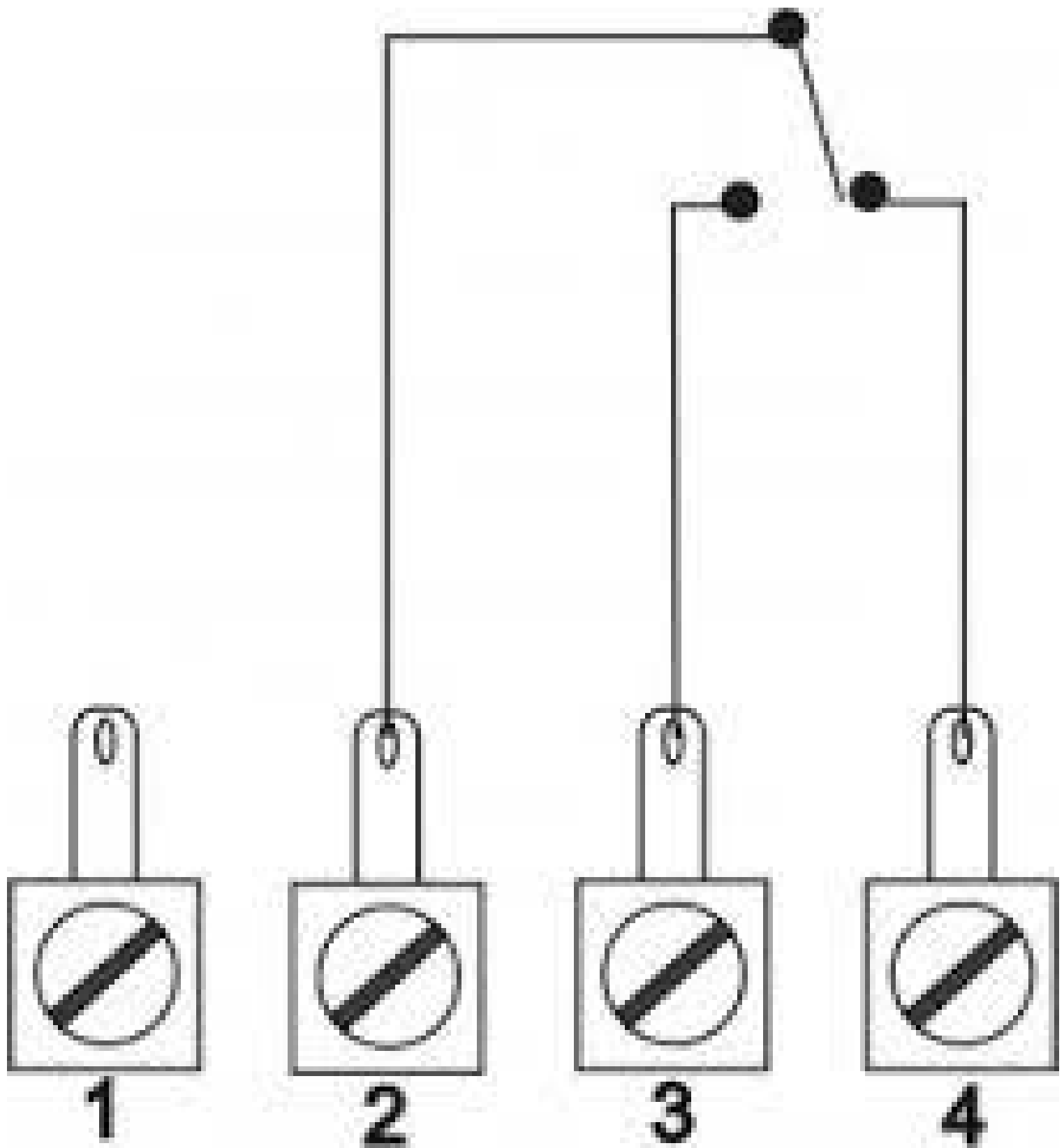
Shema spajanja PIT 92-t
